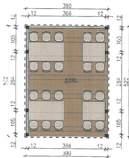
RZUT PRZYZIEMIA
