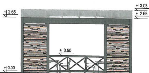
ELEWACJA BOCZNA
