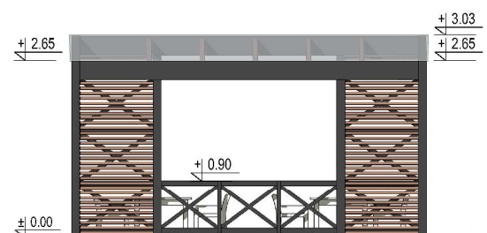
ELEWACJA BOCZNA
