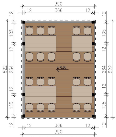
RZUT PRZYZIEMIA
